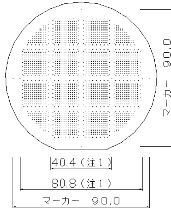
裏面 面付図 (Bottom view)
