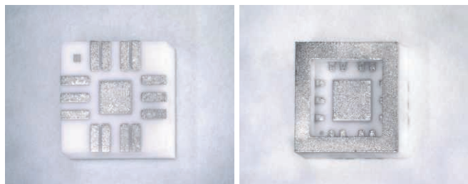
新アルミナ高温多層基板 (HTCC基板)
